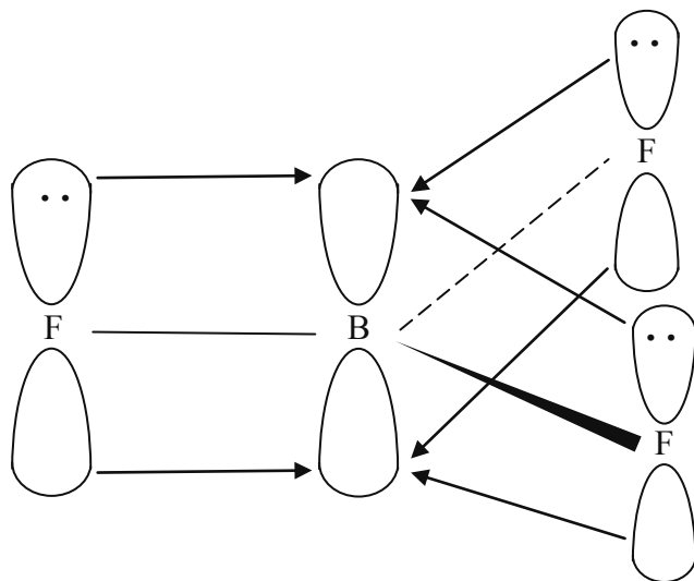
Фиг. 2. Запълване на p_z -орбиталата на В с електронна плътност от p_z -орбиталите на F-ните атоми в \text{BF}_3
