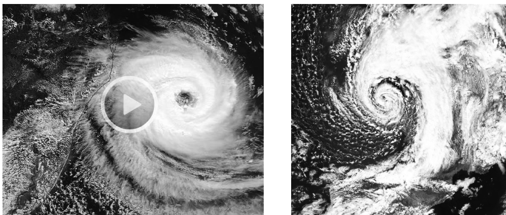
Фигура 6. Сателитна снимка на циклон над Европа според: представеното в сайта http://www.weather.com/
