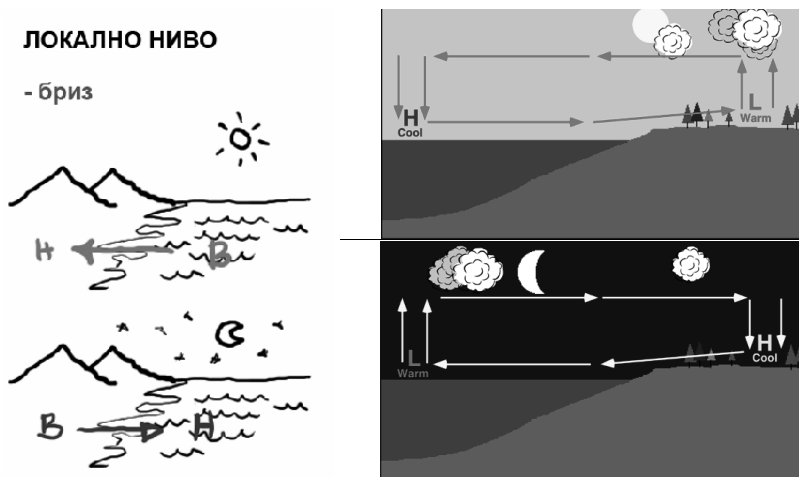
Фигура 5. Схема на въздушните течения при бризова циркулация според: представеното в сайта http://www.physicalgeography.net
