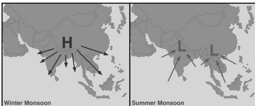
Фигура 4. Схема на мусонната циркулация над южните части на Азия http://www.physicalgeography.net/
