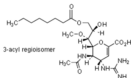
3. Oseltamivir
