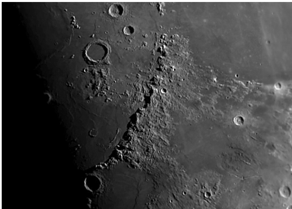
Лунните Апенини
