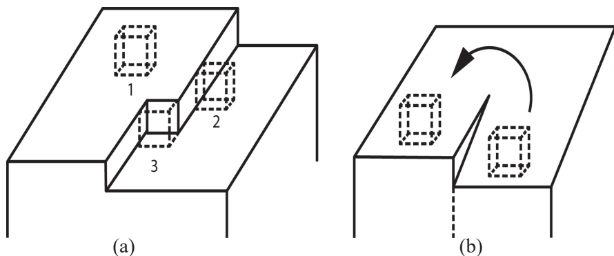
Фигура 2. Растеж на кристали: а) Молекулярно-кинетична теория на Косел (Kossel, 1927 9 ) и Странски (Stranski, 1928 8 ); б) Механизъм на винтови дислокации (Burton et al., 1951)
