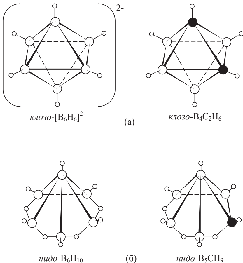
Фиг. 5. Молекулни структури на \text{closo-}[\text{B}_6\text{H}_6]^{2-} и \text{closo-B}_4\text{C}_2\text{H}_6 (а); на \text{nido-B}_6\text{H}_{10} и \text{nido-B}_5\text{CH}_9 (б)
