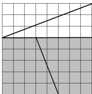
Фигура 3. Квадрат от парадокса на Фибоначи.
