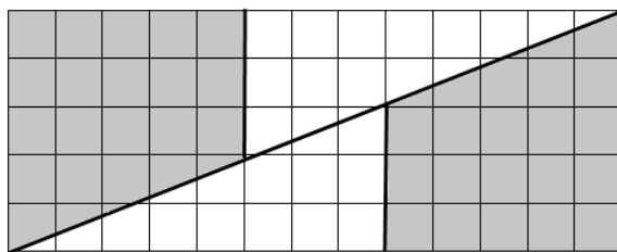
Фигура 4. Правоъгълник от парадокса на Фибоначи.
