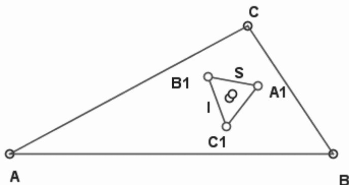
Фиг. 3. A1B1C1 е триъгълникът на de Villiers, I е центърът на вписаната окръжност в \triangle ABC , а S е точката на Малфати-Щайнер, която е изогонално-спрегнатата на I относно триъгълника на de Villiers.
