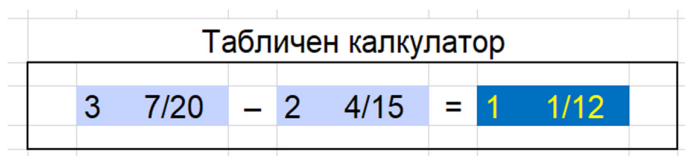
Фигура 4. Авторски табличен калкулатор в Excel за изваждане на смесени числа
