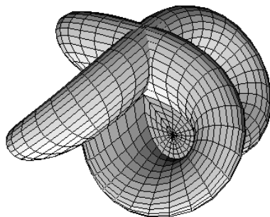
Фигура 5. Хомотопия, която извършва обръщане на сфера 6
