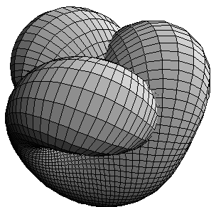
Фигура 3. Повърхнина на Бой 4
