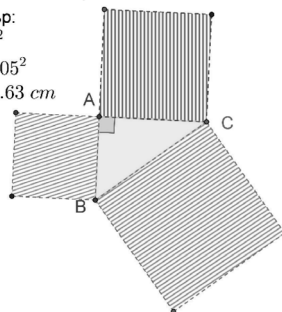
Фигура 22. Питагорова теорема със и без параметър
