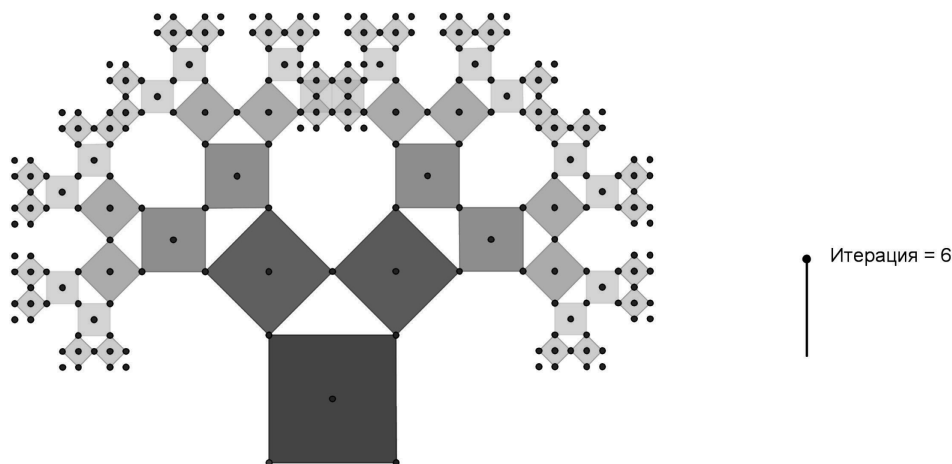
Фигура 23. Дърво на Питагор с генератор правоъгълен равнобедрен триъгълник
