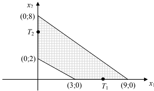
Фигура 2. Възможни положения на точките T_1 и T_2
