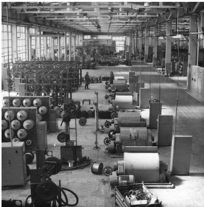
Завод за изолирани проводници, създаден през 1975 г. в гр. Смолян – производствено хале.
